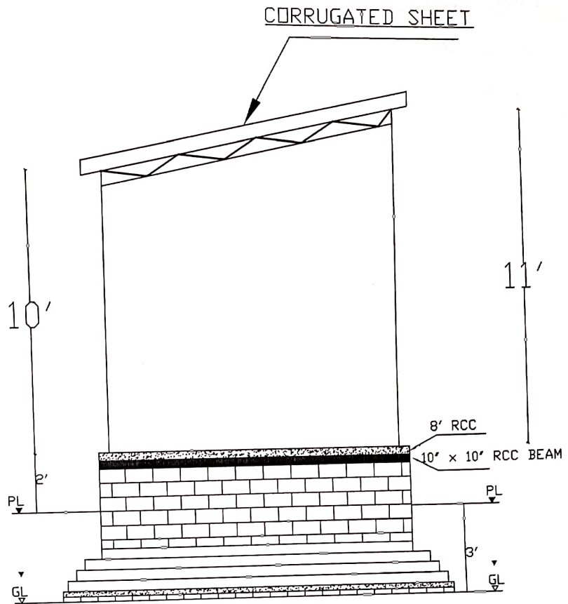
ELEVATION
